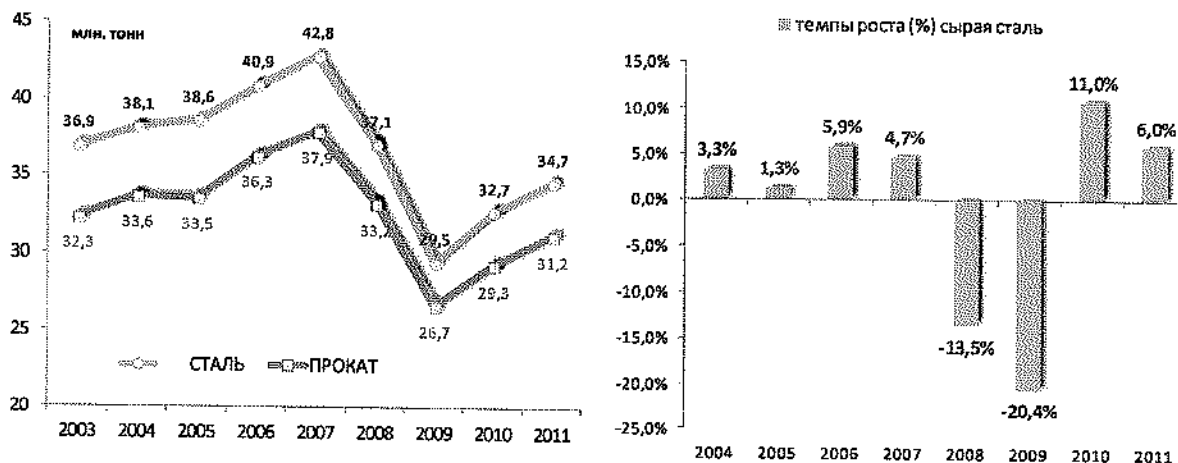
Рис. 1.1 Динамика производства стали и проката в Украине в 2003-2011 гг.
